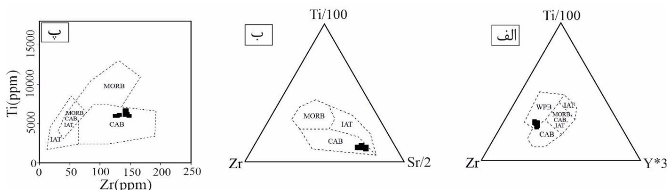
شکل ۱۰ نمودارهای شناسایی جایگاه زمین‌ساختی بازالت‌های منطقه پدران [۵۷]: (الف) نمودار سه تایی (Zr/(Ti/100)-(Y*3)؛ (ب) نمودار سه تایی (Zr/(Ti/100)-(Sr/2)؛ (پ) نمودار تغییرات Zr نسبت به Ti.
