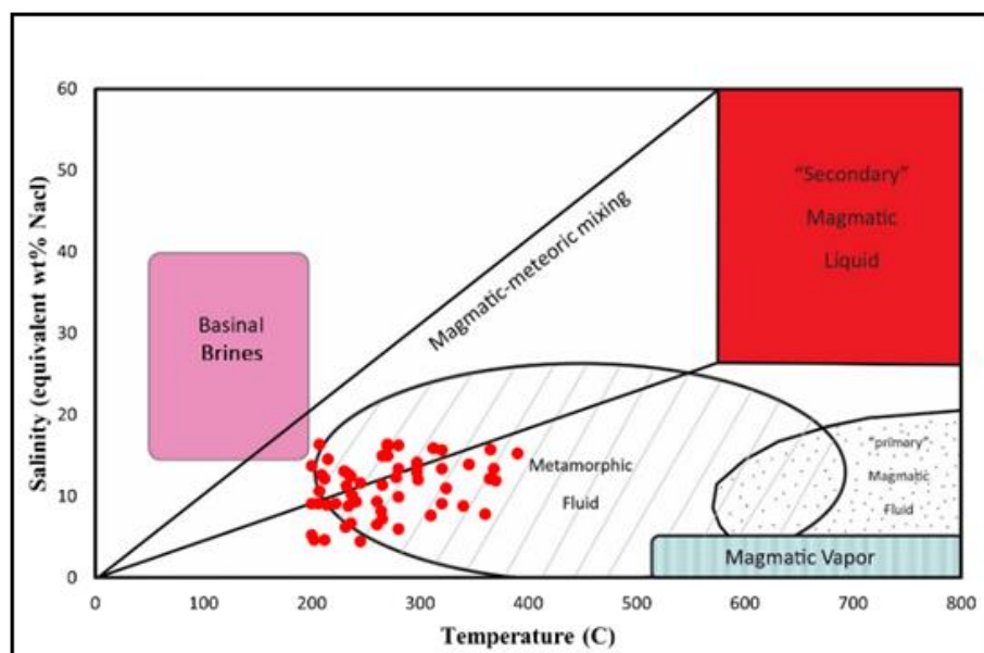
شکل ۱۰ تعیین‌کننده خاستگاه سیال کانسار ساز براساس مقدار شوری نسبت به دمای همگن‌شدگی [۳۳] که براساس آن، بیشترین تمرکز سیال‌های درگیر در منطقه در گستره آب‌های با خاستگاه دگرگونی و جوی است
