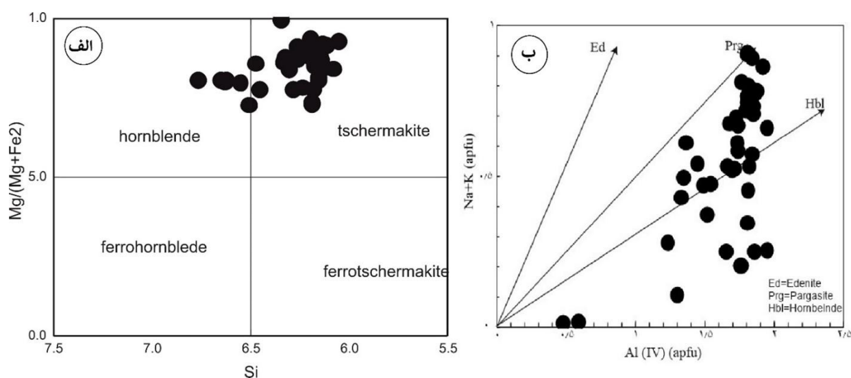
شکل ۶ الف) نمودار Si نسبت کاتیونی Mg/(Mg+Fe^{2+}) و موقعیت آمفیبول بیگانه سنگ‌های دیوریت-گابرویی در (ب) نمودار بردارهای جانشینی ادنیتی-پارگازیتی و هورنبلندی بر اساس مقادیر AlIV نسبت به (Na+K)، بیگانه سنگ‌های دیوریت-گابرویی [۱۲].
