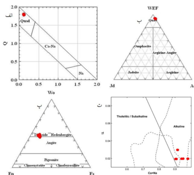
شکل ۵. الف) نمایش ترکیب پیروکسن‌های منطقه در نمودار Q-J [۱۳] (ب) نمایش ترکیب شیمیایی کلینوپیروکسن در نمودار مثلثی کوارتز-ژادئیت و آکیت [۱۳] (پ) نمایش ترکیب شیمیایی کلینوپیروکسن در نمودار مثلثی Wo-En-Fs [۱۴] (ت) استفاده از ترکیب شیمیایی کلینوپیروکسن برای تعیین سری ماگمایی [۱۴] در نمودار Ti- Ca+Na نمونه‌ها در قلمرو قلیایی قرار گرفته‌اند.
