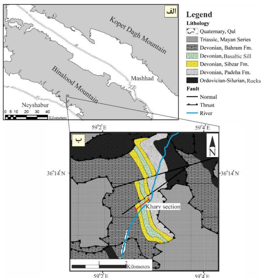
شکل ۱ الف) موقعیت مکانی سازند سبیزار در برش مورد بررسی و راه‌های دسترسی به آن، ب) بخشی از نقشه زمین‌شناسی منطقه مورد بررسی [۱۷، ۱۶].
