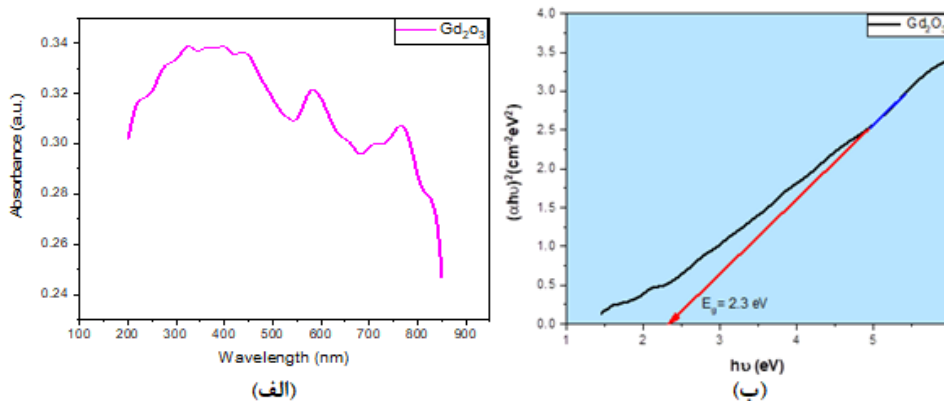
شکل ۱۴ الف) طیف جذب UV-vis اکسید گادولینیوم و ب) نمودار تاؤک برای محاسبه گاف انرژی اکسید گادولینیوم.
