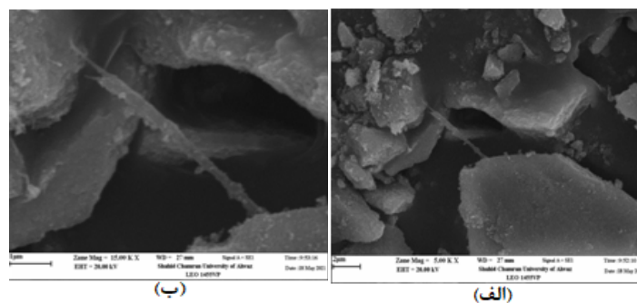
شکل ۹ تصاویر SEM نمونه دی‌اکسید تیتانیوم با ۱۱ pH در مقیاس‌های الف) ۲ میکرومتر و ب) ۱ میکرومتر.
