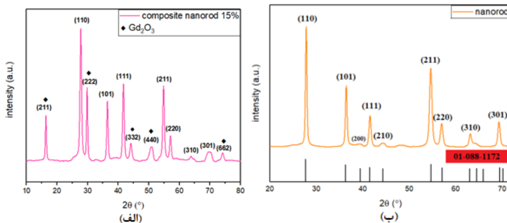
شکل ۳ مقایسه شاخص‌های میلر (الف) نانوکامپوزیت نانومیله دی‌اکسید تیتانیوم با ۱۵٪ اکسید گادولینیم و (ب) نانومیله دی‌اکسید تیتانیوم.
