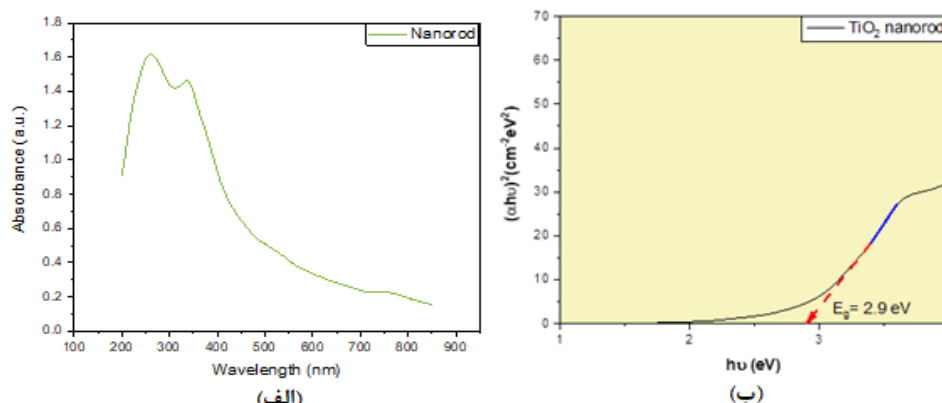
شکل ۱۵ الف) طیف جذب UV-vis نانومیله‌های دی‌اکسید تیتانیوم و ب) نمودار تاؤک برای محاسبه گاف انرژی نانومیله‌های دی‌اکسید تیتانیوم.
