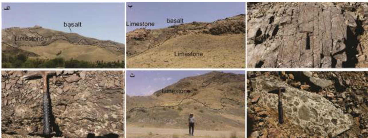
شکل ۲ الف) رخنمونی از همراهی سنگ‌های بازالتی و رسوبی منطقه مورد بررسی؛ ب) رخنمون گدازه‌های بازالتی بر روی آهک‌های کرتاسه در منطقه نوبران؛ پ) نمای نزدیک از گدازه‌های بازالتی در منطقه مورد بررسی؛ ت) کلیواژ تخته سنگی در بازالت‌های کرتاسه منطقه حلب؛ ث) رخنمونی از سنگ‌های بازالتی در قاعده سنگ‌های آهکی کرتاسه در منطقه آوج؛ ج) رخنمونی از برش‌های آتشفشانی در منطقه حلب مرز بین پهنه سندرچ- سیرجان و کمان ماگمایی ارومیه- دختر.
