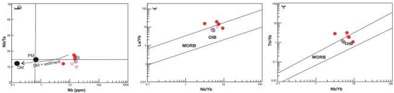
شکل ۱۰ نمودارهای الف) Nb نسبت به Nb/Ta؛ ب) و پ) Nb/Yb نسبت به M/Yb [۳۵] برای بررسی نقش اجزای فرورانش در خاستگاه سنگ‌های مورد بررسی.
