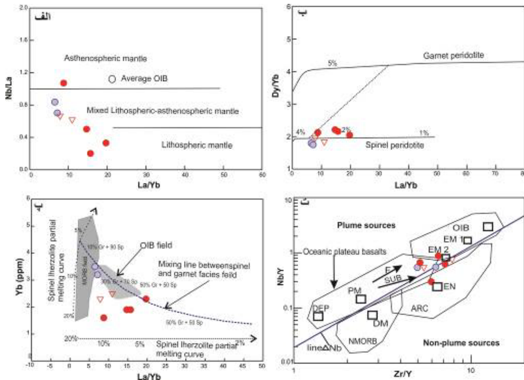
شکل ۹ نمودارهای الف) La/Yb نسبت به Nb/La [۴۶]، ب) La/Yb نسبت به Dy/Yb [۴۷]، پ) La/Yb نسبت به Zr/Y و ت) Zr/Y نسبت به Nb/Y [۴۹]، برای تعیین خاستگاه فعالیت ماگمایی در منطقه مورد بررسی. نشانه‌های استفاده شده همانند شکل ۴ هستند.
