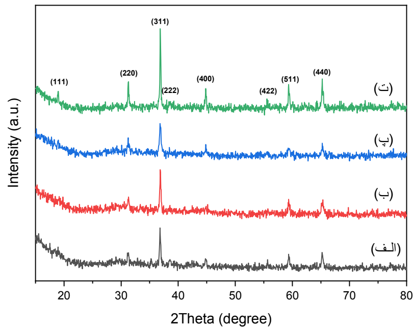
شکل ۱ طیف XRD ذرات اکسید کبالت تهیه شده به کمک لیزاب به دانه در دماهای الف) ۵۰۰، ب) ۶۰۰، پ) ۷۰۰ و ت) ۸۰۰ درجه سانتی‌گراد.
