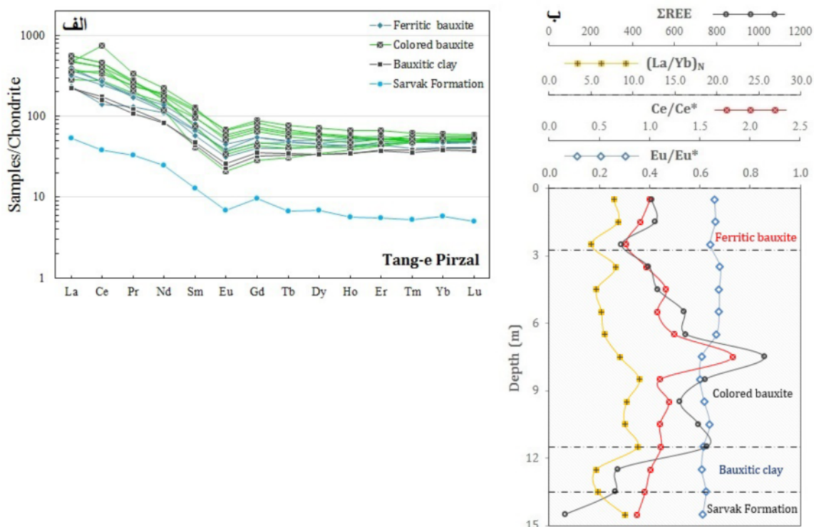
شکل ۸ الف) الگوهای عناصر خاکی نادر بهنجار شده با کندریت [۱۸]؛ ب) نمودار تغییرات شاخص‌های \text{Eu}/\text{Eu}^* , \text{Ce}/\text{Ce}^* , \text{La}/\text{Yb} و مجموع REE نسبت به عمق.
