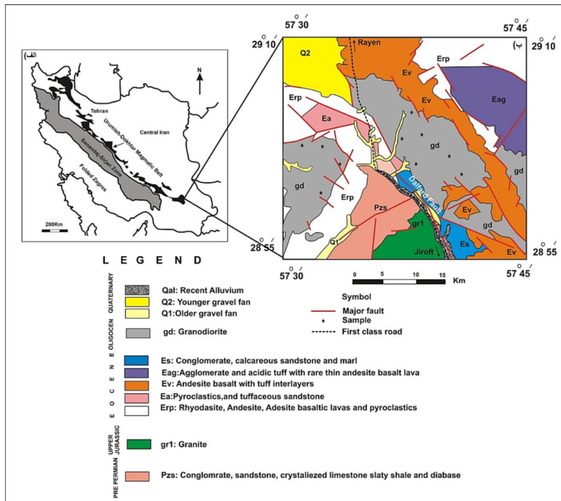
شکل ۱ الف) موقعیت منطقه مورد بررسی و کمربند ارومیه-دختر در ایران ب) نقشه ساده شده زمین شناسی منطقه مورد بررسی، برگرفته از نقشه‌های زمین شناسی ۱:۲۵۰۰۰ بم [۶،۵].
