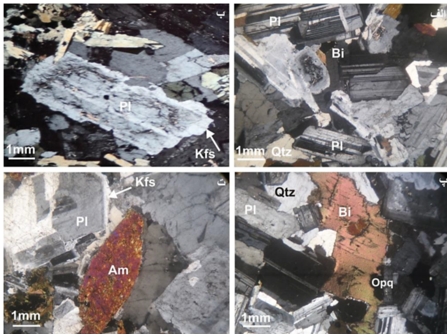
شکل ۳ الف) بافت دانه‌های ناهمسان دانه با حضور کانی‌های پلاژیوکلاز با ماکل چندریخت و منطقه بندی - بیوتیت - کوارتز در کوارتز دیوریت‌ها؛ ب) بافت آنتی راپاکیوی یا دربرگرفته شدن بلورهای پلاژیوکلاز با فلدسپات‌قلیایی در کوارتز دیوریت‌های دلفارد، پ) بلورهای بیوتیت - کوارتز در کوارتز دیوریت‌های مورد بررسی؛ ت) بلورهای آمفیبول - پلاژیوکلاز - فلدسپات‌پتاسیم - کوارتز در کوارتز دیوریت‌ها (همه تصاویر در نور قطبیده متقاطع، xpl تهیه شده‌اند).
