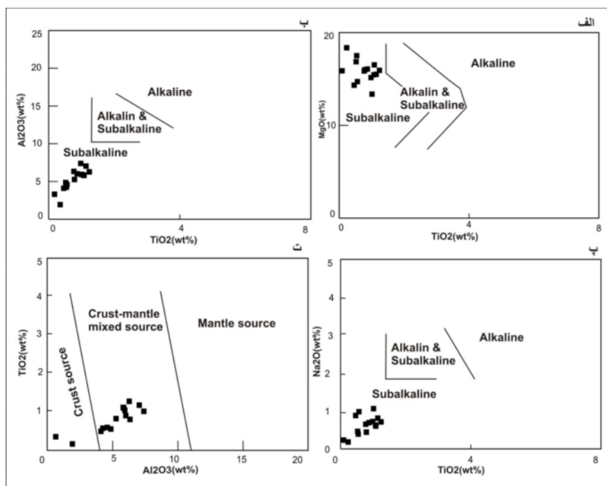
شکل ۸ الف-ب) تعیین سری ماگمایی بر اساس ترکیب شیمیایی آمفیبول [۳۲]؛ ت) نمودار Al_2O_3 نسبت به TiO_2 [۳۵] که نشان دهنده ترکیب مواد گوشته‌ای با مواد پوسته‌ای در تشکیل آمفیبول‌های مورد بررسی است.
