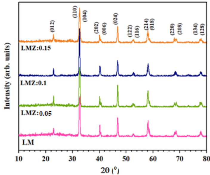
شکل ۱ الگوهای XRD نمونه‌های پروسکایت LaMn_{1-x}Zn_xO_3 ( x = 0, 0.05, 0.1, 0.15 ).
