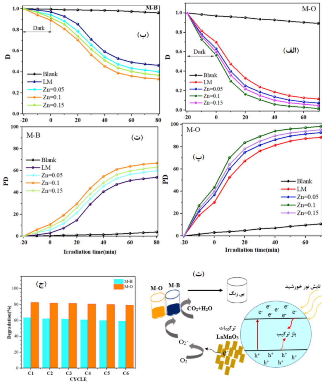
شکل ۶ (الف) و (ب) منحنی‌های تخریب، (پ) و (ت) منحنی‌های درصد تخریب محلول‌های آبی MB و MO نمونه‌های \text{LaMn}_{1-x}\text{Zn}_x\text{O}_3 ( x=0, 0.05, 0.1, 0.15 )، (ث) طرح‌های از سازوکار پیشنهادی برای تخریب فوتوکاتالیزوری و (ج) چرخه‌ی مصرف نمونه LMZ: 0.1 در تخریب دو رنگ MB و MO.
