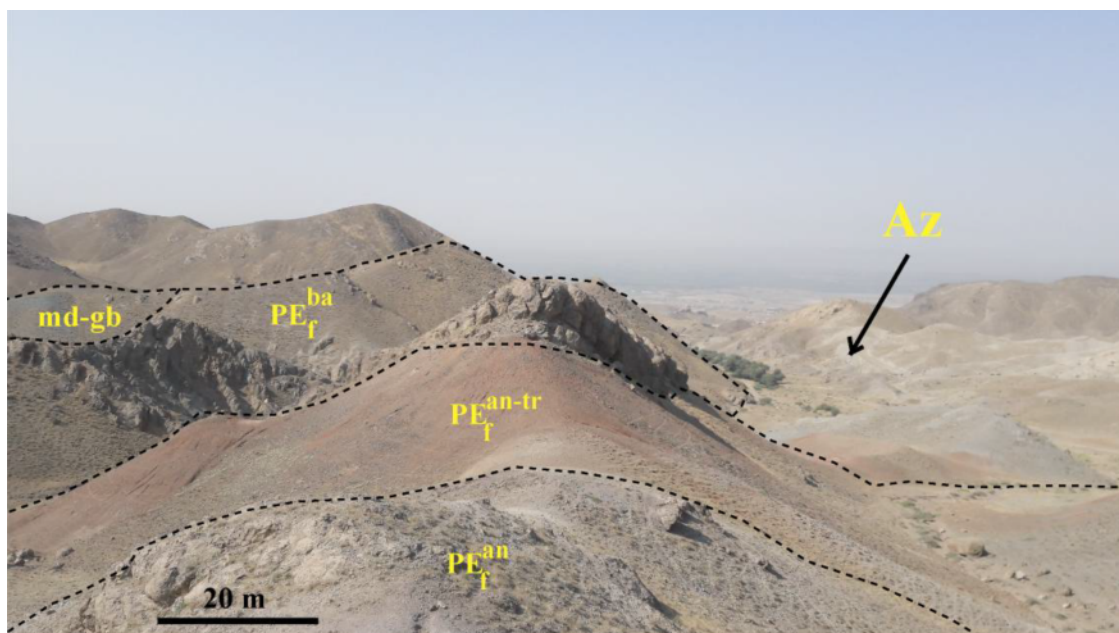
شکل ۳ نمایی از واحدهای سنگی و گسترش دگرسانی آرژلیک در گستره ذخیره مس لپه‌زنک. دید به سوی شمال. برای نشانه‌های استفاده شده بر تصویر به بخش راهنمای شکل ۲ مراجعه شود.
