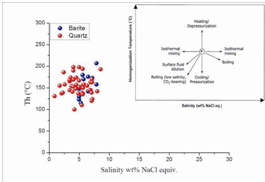
شکل ۱۱ مسیرهای توزیع میانبارهای اولیه در کانی‌های کوارتز و باریت از کانسنگ‌های مس‌دار ذخیره لپهنک در نمودار دو متغیره دمای همگن شدگی نسبت به شوری [۱۸].
