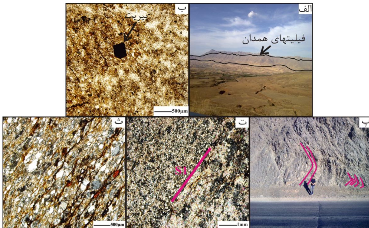
شکل ۳ الف تصویر صحرایی از فیلیته‌های همدان در شمال غرب آستانه ب: تصویر میکروسکوپی از اسلیت‌ها پ: چین‌خوردگی در شیست‌های مورد بررسی در شمال روستای چال هما ت: تصویر میکروسکوپی از شیست‌ها با فولیاسیون S1 ث: تصویر میکروسکوپی از تأثیر منطقه‌های برشی روی شیست‌های منطقه.
