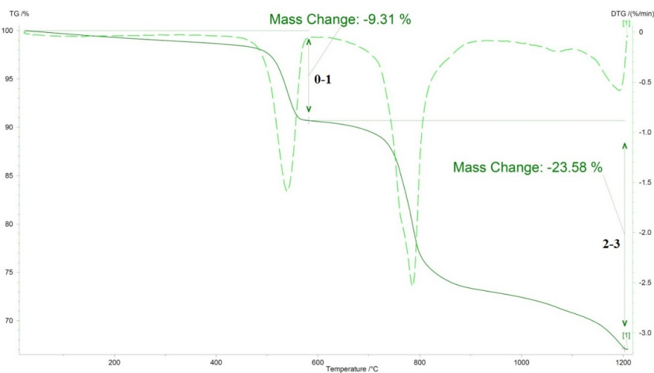
شکل ۸ نمودار گرما وزن سنجی وزنی (TGA) نمونه که دو مرحله آب‌زدایی (مرحله ۰-۱) و گوگردزایی (مرحله ۲-۳) را نشان می‌دهد.
