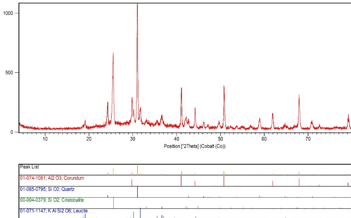
شکل ۱۱ طیف پراش پرتو ایکس نمونه پس از گرمادهی تا دمای ۱۲۰۰ درجه سانتیگراد.
