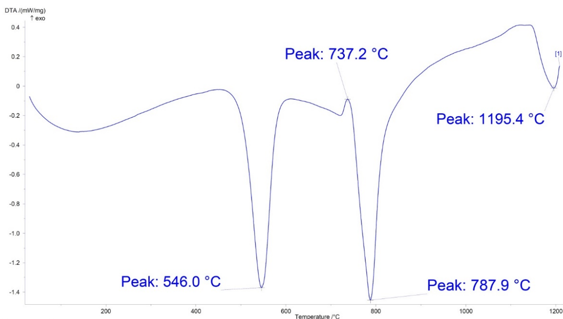
شکل ۷ نمودار گرماسنجی احتراقی (DTA) نمونه تا دمای ۱۲۰۰ درجه سانتیگراد با نرخ ۱۰ درجه بر دقیقه که نشان دهنده سه قله گرماگیر و یک قله گرماساز است.
