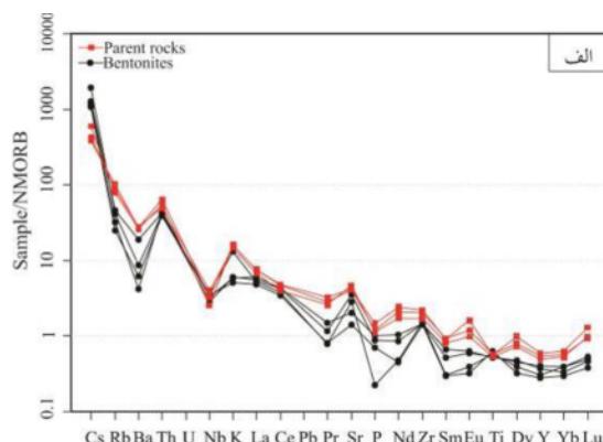
شکل ۱۰ نمودار عنکبوتی عناصر کمیاب بهنجار شده با N-MORB [۵۶]؛ ب) نمودار عناصر خاکی‌نادر بهنجار شده با کندریت [۵۷] برای گدازه‌های حدواسط و بنتونیت‌های اشکفتوک.
