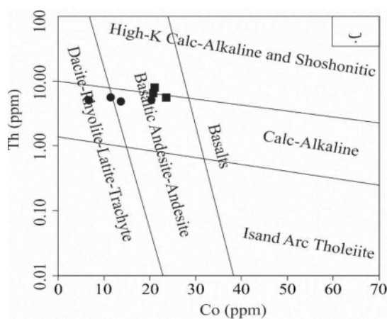
شکل ۹ نمودارهای الف) SiO 2 نسبت به Zr/TiO 2 [۵۴] و ب) Th نسبت به Co [۵۵] و موقعیت نمونه‌های بنتونیتی منطقه مورد بررسی (دایره) و سنگ مادر (مربع) بر آنها.
