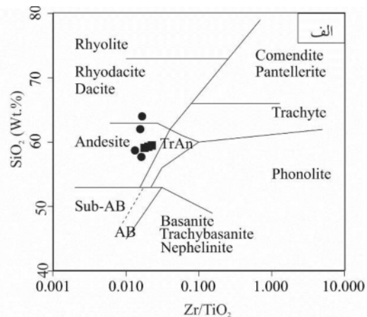
شکل ۹ نمودارهای الف) SiO 2 نسبت به Zr/TiO 2 [۵۴] و ب) Th نسبت به Co [۵۵] و موقعیت نمونه‌های بنتونیتی منطقه مورد بررسی (دایره) و سنگ مادر (مربع) بر آنها.
