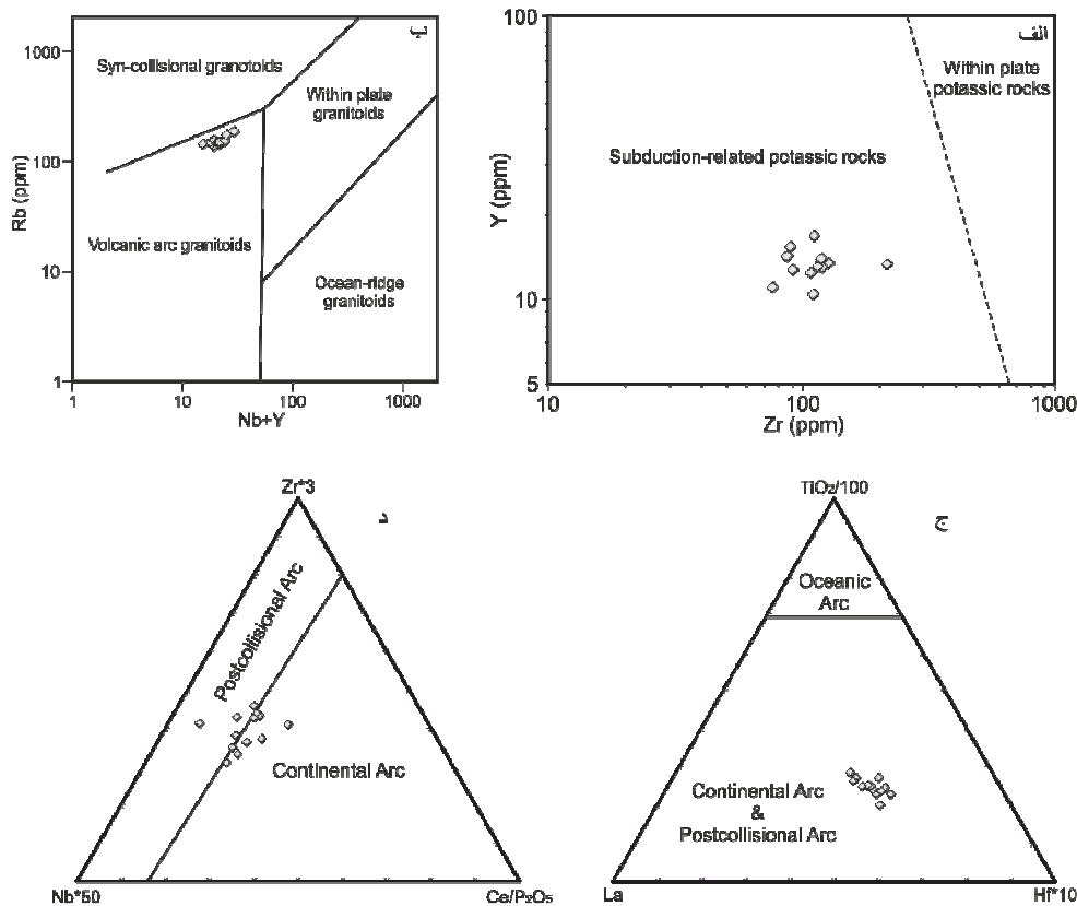
شکل ۸ الف) نمودار تغییرات Zr نسبت به Y [۳۱]؛ ب) نمودار تغییرات Rb نسبت به Nb+Y [۳۳]؛ پ) نمودار مثلثی La - TiO 2 /100 - Hf*10 [۳۲]؛ ت) نمودار مثلثی Nb*50 - Zr*3 - Ce/P 2 O 5 برای مونزونیت‌های مجموعه آذرین لار.
