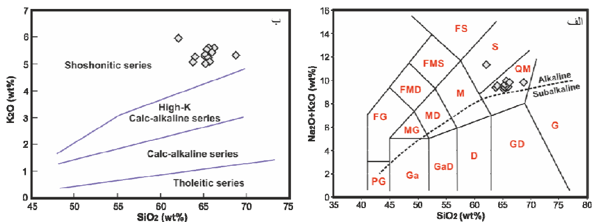
شکل ۴ الف) نمودار مجموع عناصر قلیایی نسبت به سیلیس (TAS) [۱۳]؛ ب) نمودار تغییرات K_2O نسبت به SiO_2 برای مونزونیت‌های مجموعه آذرین لار [۱۴]. (D) دیوریت، FG: فوئید گابرو، FMD: فوئید مونزودیوریت، FMS: فوئید مونزوسینیت، FS: فوئید سینیت، G: گرانیت، Ga: گابرو، GaD: گابرو-دیوریت، GD: گرانودیوریت، M: مونزونیت، MD: مونزودیوریت، MG: مونزوگابرو، PG: پریدوت گابرو و QM: کوارتزمونزونیت، S: سینیت).
