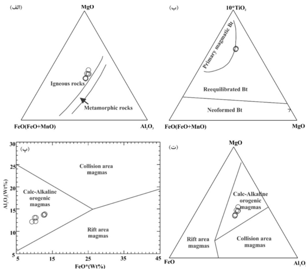
شکل ۷ تعیین ماهیت و محیط زمین ساختمانی تشکیل بیوتیت‌های موجود در دایک‌های تراکی آندزیتی ائوسن گودارسیاه (جنوب غرب جندق): (الف) نمودار مثلثی تفکیک بیوتیت‌های با ماهیت آذرین و دگرگونی [۲۴]، (ب) نمودار مثلثی تفکیک انواع بیوتیت براساس اولیه، باز تبلور یافته و یا دگرگونی بودن [۲۳]، (پ) نمودار مثلثی تقسیم بندی محیط‌های زمین ساختمانی تشکیل بیوتیت‌ها [۲۶، ۲۵] و (ت) نمودار Al_2O_3 نسبت به FeO^* برای تفکیک محیط‌های زمین ساختمانی تشکیل بیوتیت‌ها [۲۶].
