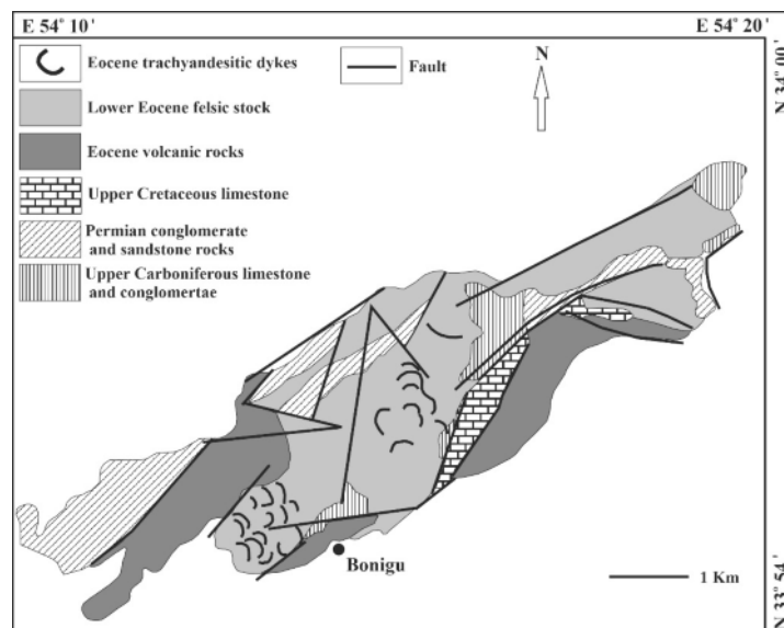
شکل ۲ نقشه زمین‌شناسی ساده شده منطقه گودارسیاه (جنوب غرب جندق) و موقعیت توده نفوذی و دایک‌های قطع‌کننده آن.
