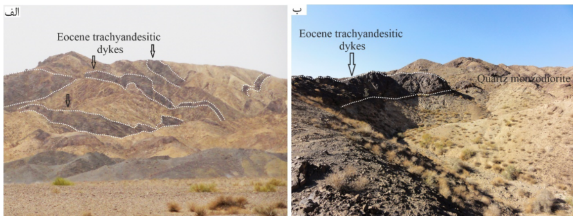
شکل ۳ تصاویر صحرایی از توده کوارتز مونزودیوریتی و دایک‌های قطع‌کننده آن در گودارسیاه (جنوب غرب جندق). (نگاه به سمت شمال).
