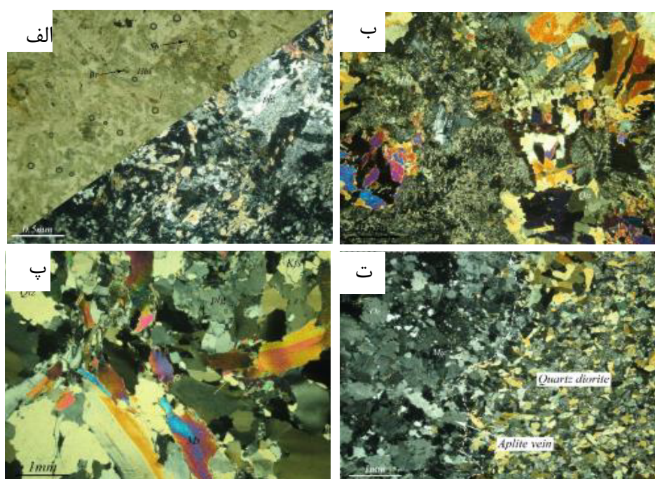
شکل ۳ تصویر میکروسکوپی از نمونه سنگ‌های منطقه مطالعاتی. الف: دیوریت با بافت دانه‌ای که در آن پلاژیوکلازها با ماکل آلبیتی و برخی از بلورهای هورنبلند دگرسان شده است (تصویر سمت چپ بالا در حالت PPL و تصویر سمت راست پایین در حالت XPL)، ب: مونزودیوریت با بافت دانه‌ای. کانی ارتوکلاز به صورت بی‌شکل در فضای بین بلورهای پلاژیوکلاز و هورنبلاند (تصویر XPL)، ج: گرانیت میلیونیتیزه. تبلور دوباره و ایجاد بافت نواری کوارتز و در لوکوگرانیت (تصویر XPL)، د: تصویر میکروسکوپی از رگه آپلیتی که در کوارتز دیوریت نفوذ نموده است. تصاویر الف و ب سمت راست تصاویر ب و ت قرار گیرند.
