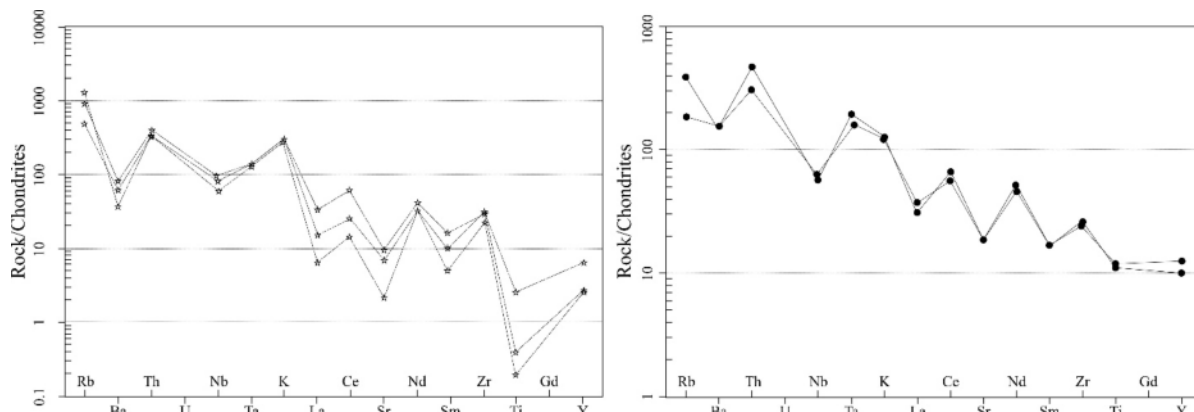
شکل ۹ نمودارهای عناصر خاکی نادر سنگ‌های منطقه باغچه‌مریم به‌نچارشده نسبت به کندریت [۲۴] (نشانه * : سنگ‌های اسیدی و ● : سنگ‌های حدواسط).
