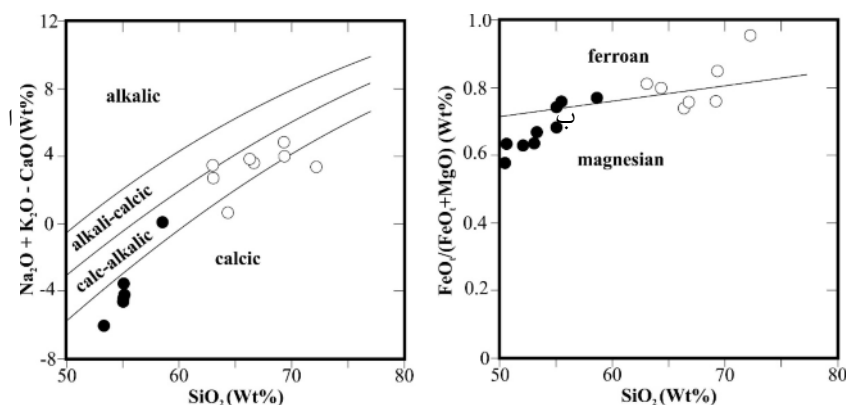
شکل ۶ الف) نمودار \text{SiO}_2 نسبت به (\text{Na}_2\text{O} + \text{K}_2\text{O} - \text{CaO}) [۱۷] و ب) نمودار \text{SiO}_2 نسبت به (\text{FeO}/(\text{FeO} + \text{MgO})) [۱۷] و موقعیت نمونه‌های مورد بررسی بر آن‌ها (دایره تو خالی: سنگ‌های اسیدی و دایره توپر: سنگ‌های حدواسط). تصویر الف سمت راست تصویر ب قرار گیرد.
