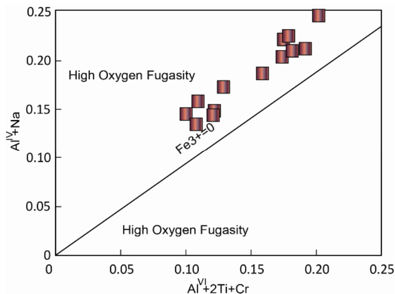
شکل ۷ موقعیت کلینوپیروکسن‌های نمونه‌های آذرین جنوب آزادشهر در نمودار تغییرات گریزندگی اکسیژن براساس \text{Al}^{\text{IV}} + \text{Na} نسبت به \text{Al}^{\text{VI}} + 2\text{Ti} + \text{Cr} در پیروکسن‌ها [۳۴].
