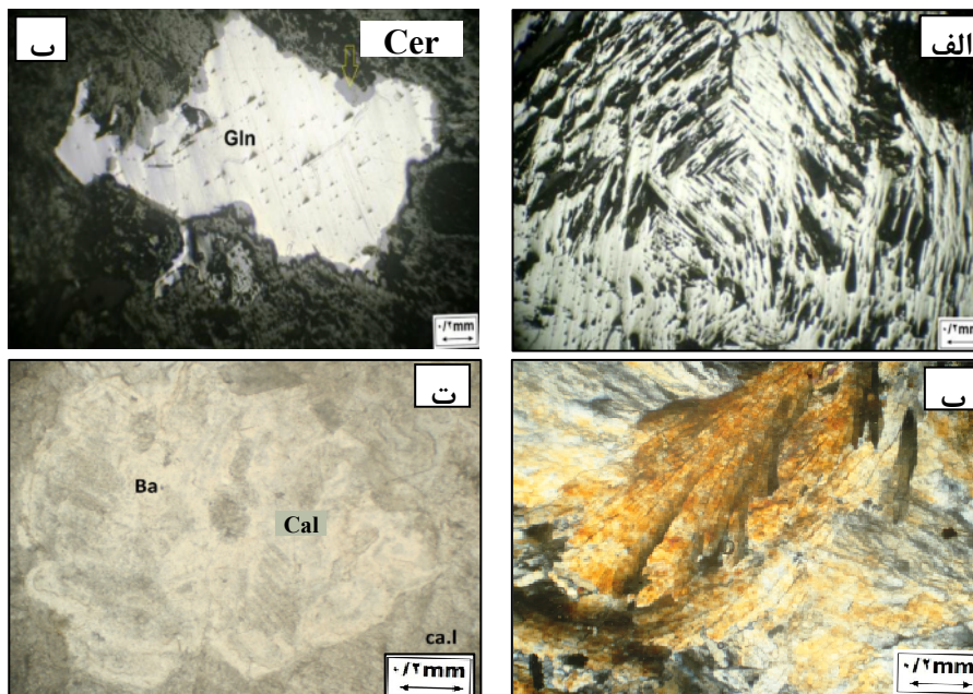
شکل ۴ تصاویر میکروسکوپی از الف) گالن با رخ شمشیری (XPL)، ب) تبدیل گالن (Gln) در لبه‌ها به سروزیت (Cer)، پ) باریت با بافت پرماند و ماکل تکراری (XPL) و ت) حضور باریت (Ba) در زمینه کلسیت (Cal) (PPL). (نشانه‌های اختصاری بر گرفته از مرجع [۲۵] هستند).
