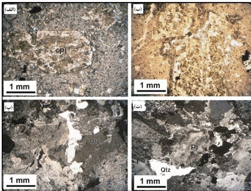
شکل ۸ تصاویر میکروسکوپی از گرانیت پورفیری: الف) درشت بلورهای پلاژیوکلاز (Pl) که بطور بخشی توسط سریسیت جایگزین شده‌اند، ب) سریسیتی‌شدگی سنگ، پ و ت) جایگاه بین دانه‌ای و بی‌شکل کوارتز (Qtz) بین بلورهای پلاژیوکلاز (Pl).
