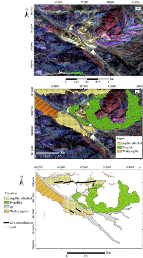
شکل ۴ الف) تصویر ماهواره‌ای پردازش‌شده از منطقه مورد بررسی که روند خطی دگرسانی آرزیلی منطبق برکانی‌سازی (به ویژه در شمال منطقه) مشهود است، ب) تطبیق نقشه دگرسانی بر تصویر ماهواره‌ای و پ) نقشه دگرسانی و کانی‌سازی در منطقه بیدوک.
