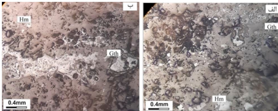
شکل ۷ کانی‌سازی بصورت الف) پراکنده و ب) رگه‌ای (نور XPL) که به اکسیدها و هیدروکسیدهای آهن دگرسان شده اند. (Hm: هماتیت و Gth: گوتیت از [۱۵]).
