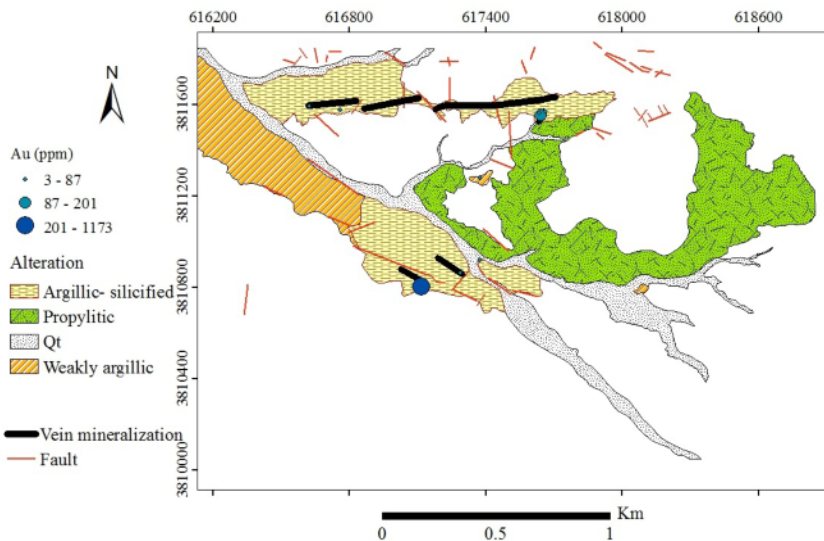
شکل ۸ نقشه پراکنده‌گی زمین‌شیمیایی عنصر طلا در منطقه مورد بررسی. جدول ۲ ضریب همبستگی عناصر در منطقه بیدوک (سطح اطمینان ۰,۰۵ است).
