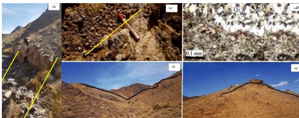
شکل ۵ الف) مقطعی از رگه سیلیسی که در لبه به کانی‌های رسی دگرسان شده است (نور XPL). ب) دگرسانی آرژیلی در لبه رگه سیلیسی- اکسید آهن، پ و ت) رخنمون رگه‌های سیلیسی- اکسید آهنی با روند شمال‌غرب- جنوب‌شرقی در منطقه بیدوک (دید به سمت شرق)، ث) راستای رگه سیلیسی (خطوط زرد) منطبق بر سطح گسل که در کف آبراهه رخنمون یافته است. (دید عکس به سمت شمال). (Qz): کوارتز [۱۵]
