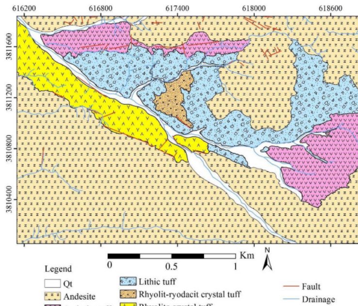
شکل ۳ نقشه زمین‌شناسی منطقه بیدوک.
