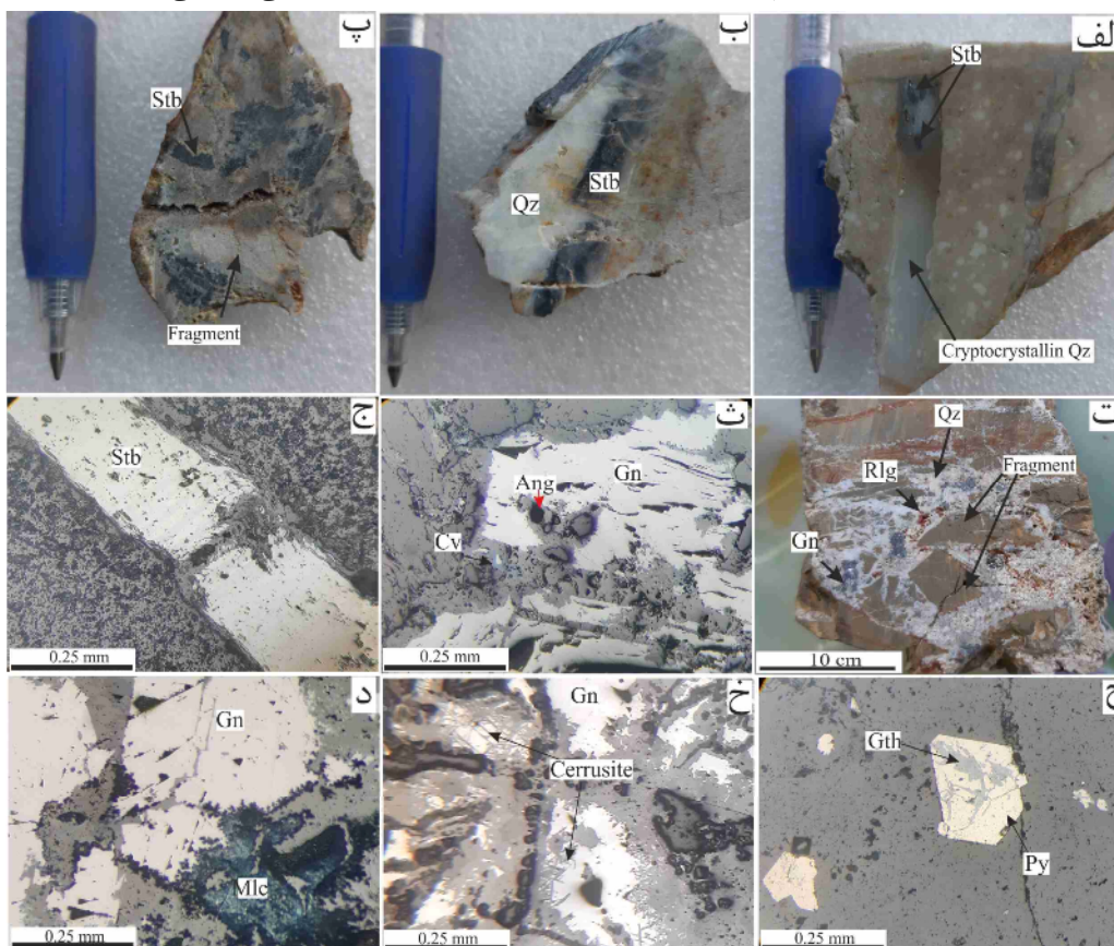
شکل ۴ نمونه دستی از کانی‌سازی در منطقه کوه شور و تصاویر میکروسکوپی در نور بازتابی از الف) رگچه‌های کوارتز نهان بلوری-استینیت در واحد داسیتی، ب) رگه کوارتز-استینیت در واحد داسیتی، پ) استینیت-کوارتز نهان بلوری در برش گسلی با قطعه‌هایی از سنگ میزبان داسیتی. ت) گالن-زرنیخ قرمز-کوارتز در برش گسلی با قطعه‌هایی از واحد شیلی، ث) گالن از لبه در حال تبدیل به آنگلیت (PPL)، ج) ستون‌های کشیده استینیت (PPL)، ح) پیریت بیشتر به صورت شکل‌دار تا نیمه شکل‌دار در حال تبدیل به گوتیت (PPL)، خ) تبدیل گالن به سروزیت (PPL)، د) ملاکیت (PPL). پیریت، Py = پیریت، استینیت، St = استینیت، Ang = آنگلیت، Gn = گالن، Cv = کوولیت، Gth = گوتیت، Rlg = زرنیخ قرمز، Qz = کوارتز و Mlc = ملاکیت [۱۳].
