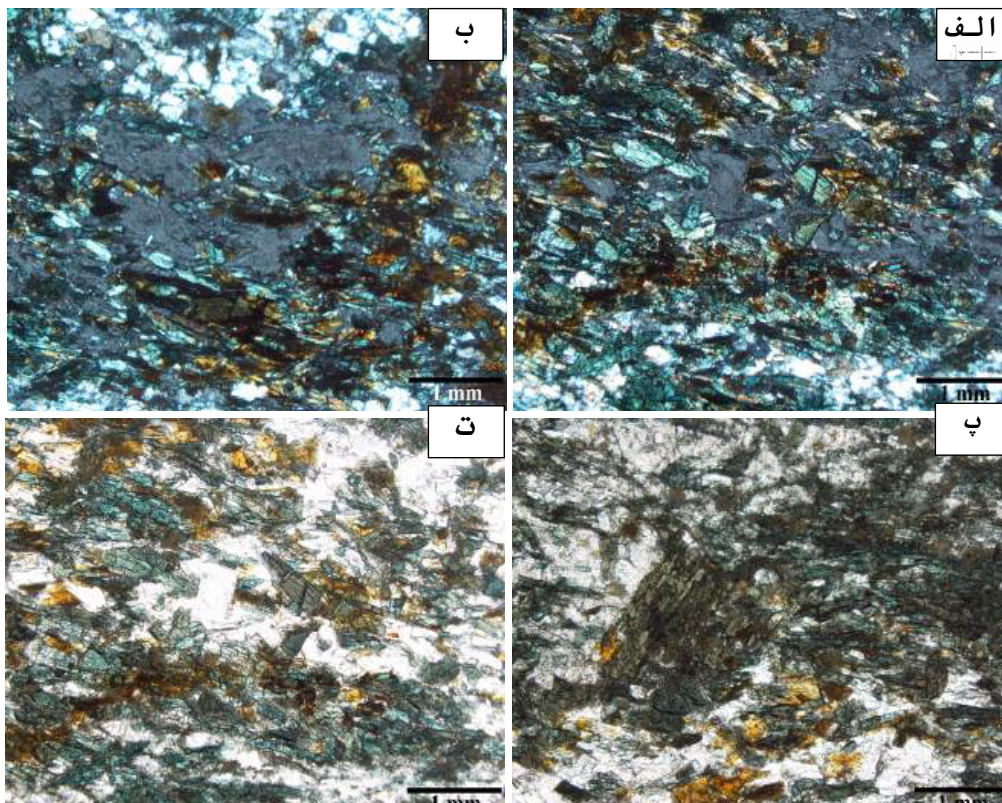
شکل ۳ تصاویر میکروسکوپی از شیبست‌های مورد بررسی نشان دهنده: (الف) بافت غالب پورفیری غربالی ورقه‌نح شکفتی و مجموعه کانیایی آمفیبول، آلبیت، موسکوویت و کلریت در نور دو بار قطبیده؛ (ب) پورفیری غربالی‌های آلبیتی با میانبرهایی از آمفیبول و دارای لبه فشارشی از کلریت و موسکوویت در نور دوبار قطبیده؛ (پ) شکفته بلورهای آمفیبول مایل نسبت به شیبستوارگی اصلی و تبدیل‌شدگی به کلریت از لبه در نور یک بار قطبیده؛ (ت) آمفیبول‌های موجود در راستای شیبستوارگی اصلی با ساختار منطقه‌بندی در نور یک بار قطبیده. نام‌های اختصاری کانی‌ها: Chl: کلریت، Amp: آمفیبول، Ab: آلبیت و Ms: موسکوویت) برگرفته از مرجع [۱۵] است.
