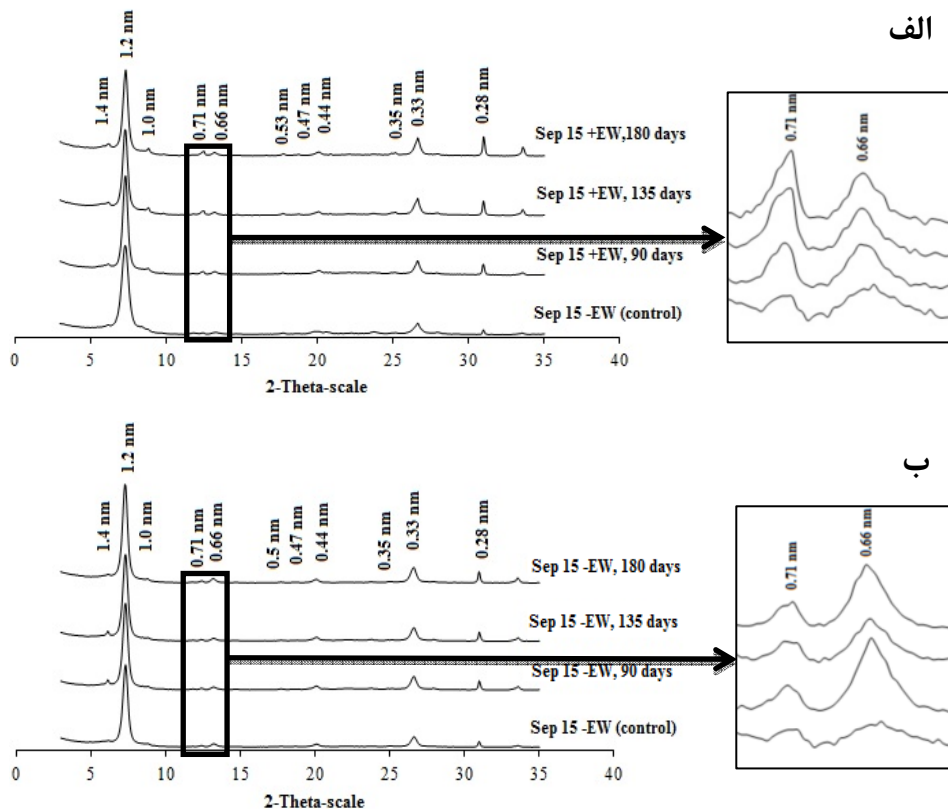
شکل ۲ پراش نگاشت‌های پرتوی ایکس از نمونه‌های منیزیم-اشباع (Mg) تیمارهای دارای سپیولیت و فرآورده‌های هوادیدگی احتمالی آن در زمان‌های مختلف نمونه‌برداری و در شرایط با (الف) و بدون (ب) کرم خاکی در مقایسه با نمونه شاهد (کنترل).
