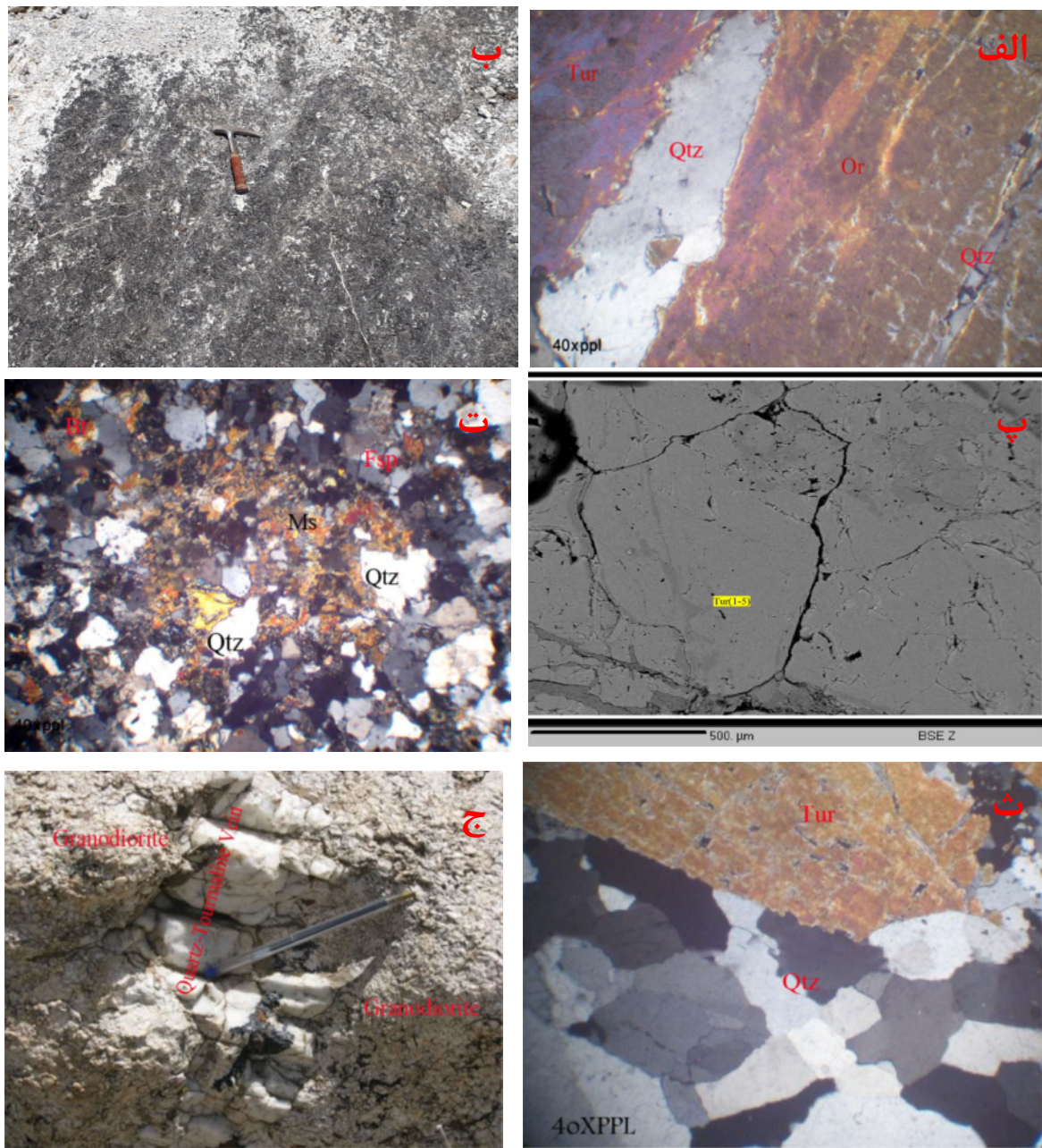
شکل ۳ تصاویر صحرایی، میکروسکوپی و ریزپردازش الکترونی واحدهای تورمالین‌دار: (الف) تصویر میکروسکوپی از پگماتیت تورمالین‌دار با بافت پگماتوئیدی، (ب) تصویر صحرایی از تورمالین به طول تقریبی ۱۴ تا ۲۲ میلی‌متر و پگماتیت‌های موجود در توده‌های گرانیتوئیدی (دید به سمت جنوب). (پ) تصویر ریزپردازش الکترونی از تورمالین‌های موجود در پگماتیت‌ها، (ت) تصویر میکروسکوپی از واحد گرانودیوریت با بافت دانه‌ای و شامل کانی‌های کوارتز، پلاژیوکلاز، فلدسپات قلیایی، بیوتیت و موسکویت، (ث) تصویر میکروسکوپی از فلدسپات و تورمالین موجود در رگه‌های کوارتز-تورمالین. (ج) رگه‌های کوارتز-تورمالین در سنگ‌های گرانودیوریتی (دید به سمت شرق). (Qtz): کوارتز- Hbl: هورنبلند، -Fsp: فلدسپار، -Pl: پلاژیوکلاز، -Mc: میکروکلین، -Bt: بیوتیت، -Ms: موسکوویت، -Or: ارتوز-و-Tur: تورمالین [۴۰].
