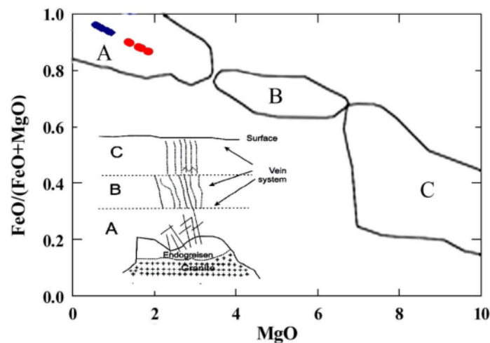
شکل ۷ نمودار FeO^{*} = FeO / (FeO + MgO) نسبت به MgO که در آن، میدان تورمالین‌های اندوگرانیته تا نزدیک به توده گرانیتی (A)، نزدیک به توده گرانیتی تا حدواسط (B) و تورمالین‌های دور از توده گرانیتی (C) مشخص شده است [۵۱]. همه نمونه‌های برداشت شده از تورمالین‌های منطقه مالمیر در گستره A واقع هستند. نشانه‌ها مانند جدول ۱ هستند.
