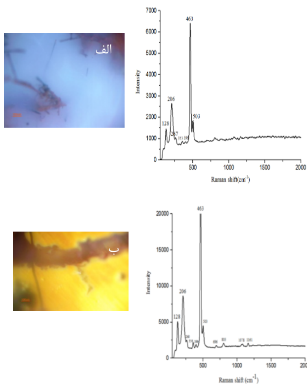
شکل ۱۱ الف . تصاویر میکروسکوپی و طیف‌های رامان کوارتز، موگانیت و همتایت در ژاسپ‌های شاخه ای الف) خاکستری و ب. زردرنگ
