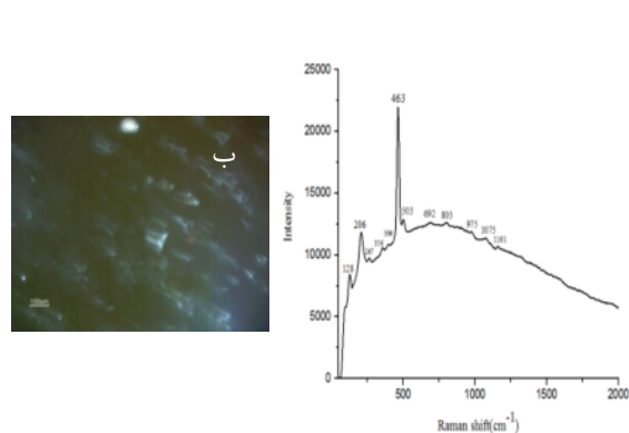
شکل ۷ الف. تصویر میکروسکوپی و طیف‌های رامان الف) کوارتز، موگانیت و مواد کربن‌دار در آگات-ژاسپرهای استالاکتیتی قرمز و سبز. و ب) کلریت در آگات-ژاسپرهای استالاکتیتی قرمز و سبز.
