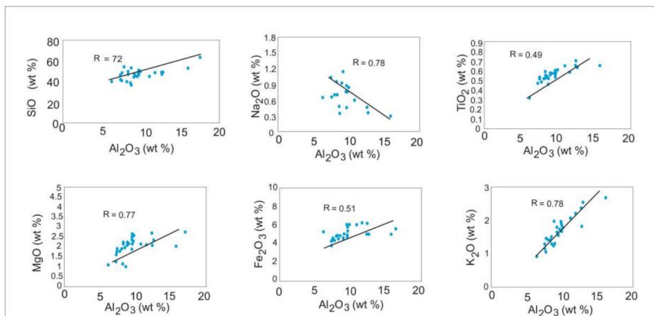
شکل ۸. نمودارهای پراکندگی تغییرات اکسیدهای اصلی نسبت به \text{Al}_2\text{O}_3 در شیل‌های منطقه.
