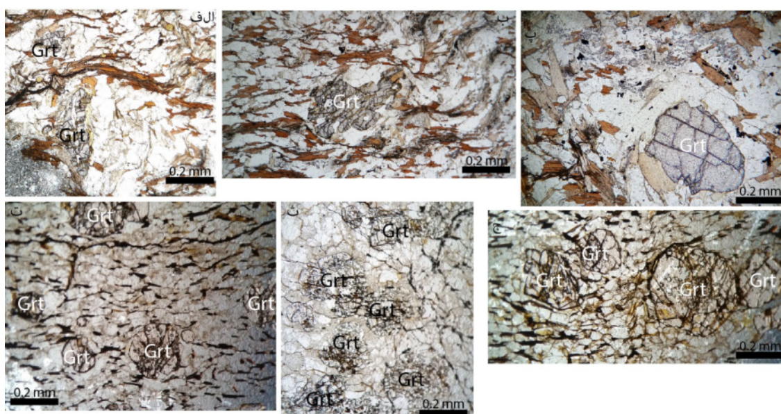
شکل ۵ تصاویر میکروسکوپی از شیبست‌های گارنت‌دار شاهیندژ (SMC) بصورت منفرد در متن جهت‌یافته سنگ.
