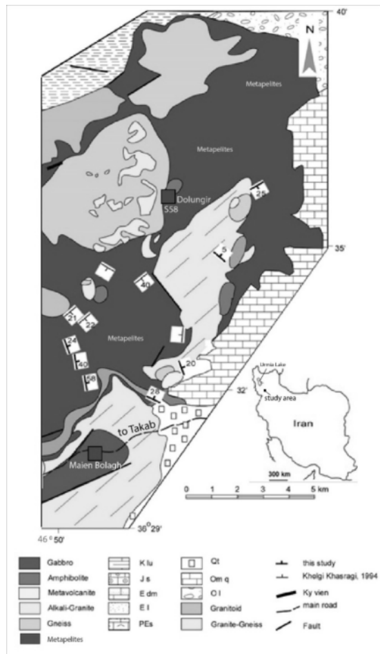
شکل ۱ نقشه زمین‌شناسی از منطقه همتافت دگرگونی شاهیندژ (SMC) در جنوب آذربایجان غربی [۳۰].
