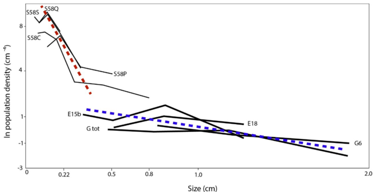
شکل ۱۰ مقایسه الگوی CSD گارنت‌های شیست‌های شاهیندژ (خطوط سیاه نازک) با هورنفلس‌های دوربه (خطوط سیاه پر رنگ). شیب خط وایزش چشمی برای شیست‌های شاهیندژ با خط چین قرمز و برای هورنفلس‌های دوربه با خط چین آبی نشان داده شده است.
