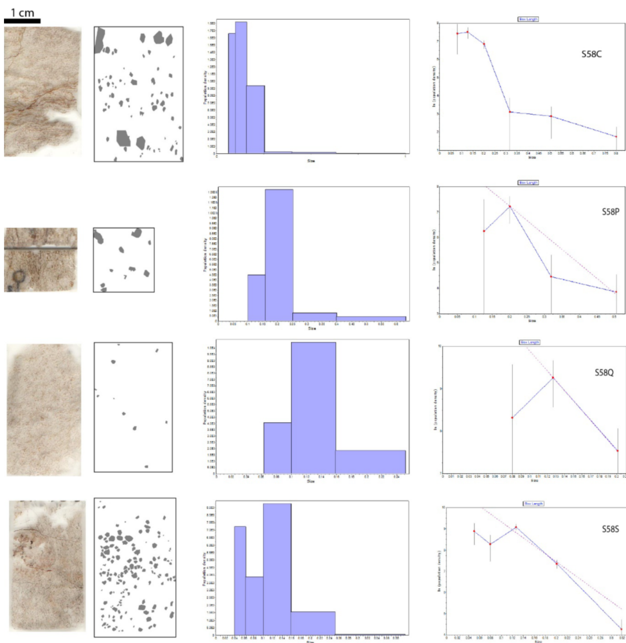
شکل ۸ طرحواره مقاطع نازک از شکفته بلورهای گارنت، نمودار تجمعی ستونی برای دانه‌های گارنت و نیز نمودار توزیع ابعاد بلوری برای گارنت-های موجود در شیت‌های شاهیندژ (SMC).
