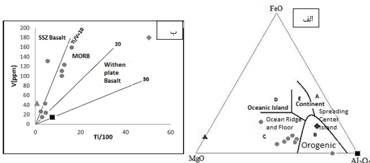
شکل ۱۵ الف: نمودار Al_2O_3 و FeO و MgO جهت تعیین محیط زمین ساختی از [۲۹]. ب: نمودار V در مقابل [Ti/100] که بیشتر نمونه‌ها در گستره بازالت‌های پشته میان اقیانوسی قرار دارند.
