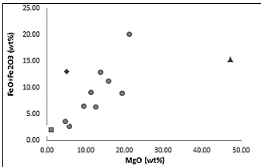
شکل ۲۱ نمودار تغییرات \text{FeO}+\text{Fe}_2\text{O}_3 نسبت به \text{MgO} برای سنگ‌های منطقه مورد بررسی که نشان دهنده تهی‌شدگی آهن در مراحل اولیه جدایش است.
