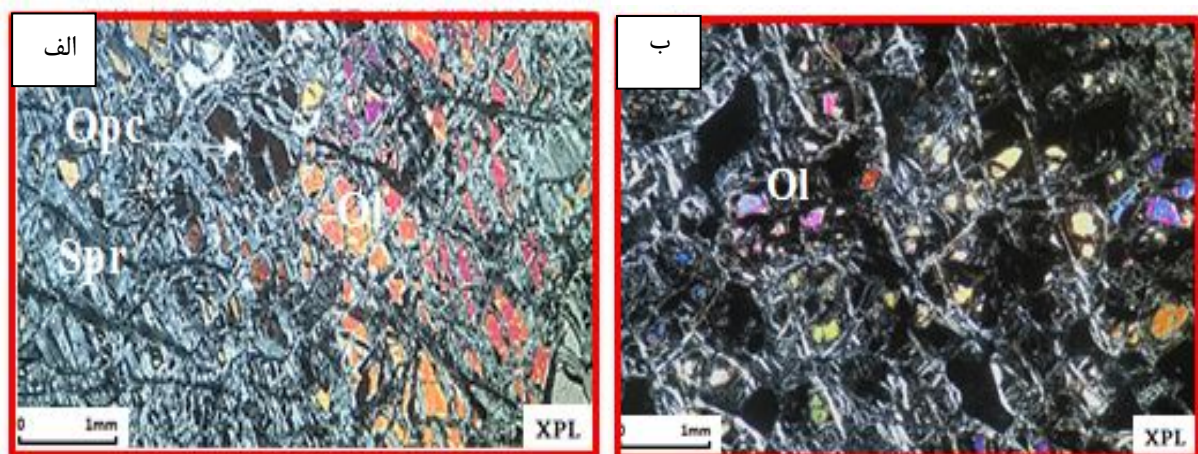
شکل ۱۰ تصاویری میکروسکوپی از لرزولیت‌های مجموعه افیولیتی شرق دشت سمسور: الف) وجود کانی‌های اولیوین (Ol)، کدر (Opc) و سرپانتین (Spr) در سنگ که حجم بیشتر سنگ را اولیوین تشکیل داده، در حال تجزیه به سرپانتین بوده و باعث ایجاد، بافت شبکه‌ای گردیده است، ب) وجود حجم بالای کانی آپیک در بین کانی‌های اولیوین (Ol) و سرپانتین (Spr) (همه تصاویر در نور قطبیده متقاطع، XPL، با بزرگ‌نمایی 40X تهیه شده‌اند).
