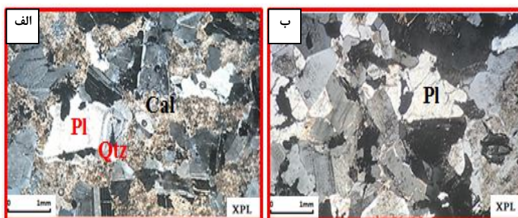
شکل ۱۱ تصاویری میکروسکوپی از پلاژیوگرنیت‌های مجموعه افیولیتی شرق دشت سمسور: الف) درشت بلور پلاژیوکلاز (Pl) با ماکل شاخص چندریخت همراه با کوارتز (Qtz) دانه ریز در زمینه، هورنبلند (Hlb) و پلاژیوکلازهای در حال دگرسان شدن به کلسیت (Cal). ب) بلورهای دانه درشت پلاژیوکلاز (Pl) به نسبت سالم با ماکل چندریخت همراه با مقدار کمی کلریت (Chl) در زمینه سنگ (همه تصاویر در نور قطبیده متقاطع، XPL، با بزرگ‌نمای 40X تهیه شده‌اند).
