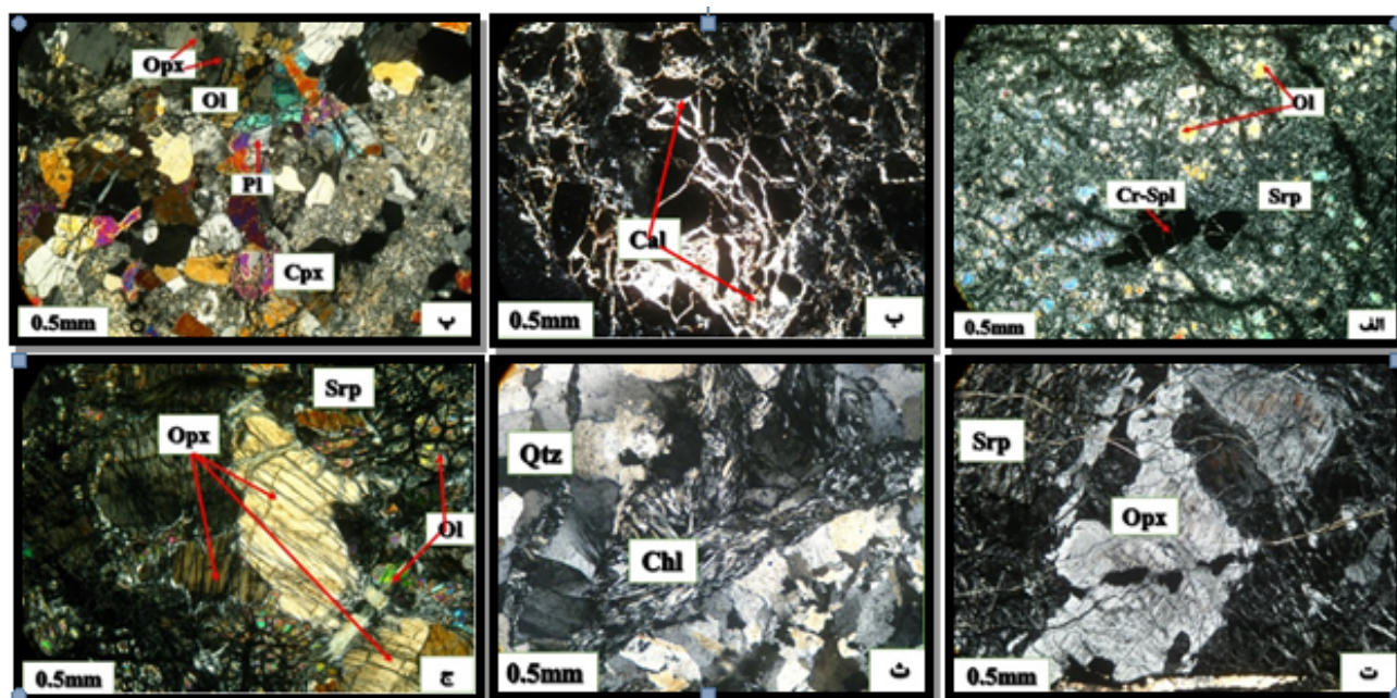
شکل ۶ تصاویر میکروسکوپی از سنگ‌های الترامافیک منطقه‌ی شرق سریش: الف) سربانتینیت‌ها به همراه آثاری از کانی‌های الیوین (Ol)، اسپینل کروم‌دار (Cr-Spl) و سربانتین (Srp) و کانی‌های کدر با بافت مشبک، ب) حضور کانی‌های ثانویه‌ی کلسیت (Cal) و اکسیدهای آهن در سنگ به همراه بافت برشی، پ) سنگ الیوین گابرو حاوی کانی‌های پلاژیوکلاز (Pl)، الیوین (Ol)، ارتوپروکسن (Opx) و کلینوپروکسن (Cpx)، ت) ارتوپروکسن نوع برنزیتی که باستیتی شده است (Qtz) و کلریت دم گریه‌ای (Chl)، ج) هارزبورژیت به همراه کانی‌های الیوین، ارتوپروکسن و سربانتین (تمامی تصاویر در نور XPL تهیه شده‌اند). کوتاه نوشت کانی‌ها [ ۹ ].
