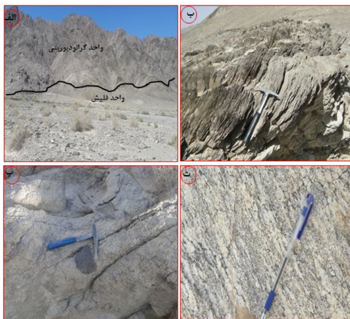
شکل ۳ الف: نمایی از مرز بین واحدهای گرانیتی کوه ریگ ملک با سنگ‌های میزبان فلیشی (دید جنوب شرقی)، ب- نمایی نزدیک از واحدهای اسلیت و فیلیت منطقه کوه ریگ ملک (جهت دید جنوب شرقی)، پ- ساختار میلونیتی و نواری در گرانیت میلونیتی شده کوه ریگ ملک. ت- برونوم تیره رنگ (متاپلیتی) موجود در واحدهای گرانیتی.
