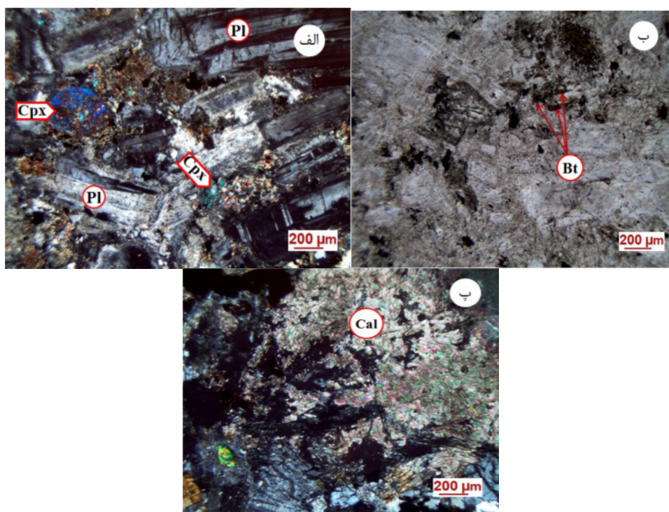
شکل ۲ تصاویر میکروسکوپی سنگ میزبان رگه‌های کوارتز (الف) نمایی از بافت دانه‌ای در کوارتز مونوزودیوریت، پیروکسن (Cpx) با لبه‌های نیمه گرد شده و بلورهای درشت پلاژیوکلاز رسی شده در نور قطبیده متقاطع (XPL)، (ب) کانی بیوتیت (Bt) ثانویه بصورت پراکنده در نور قطبیده صفحه‌ای (PPL) و (پ) تشکیل کانی کلسیت (Cal) در بخش‌هایی از سنگ میزبان در نور XPL. علائم اختصاری کانی‌ها برگرفته از مرجع [۲۴] است.
