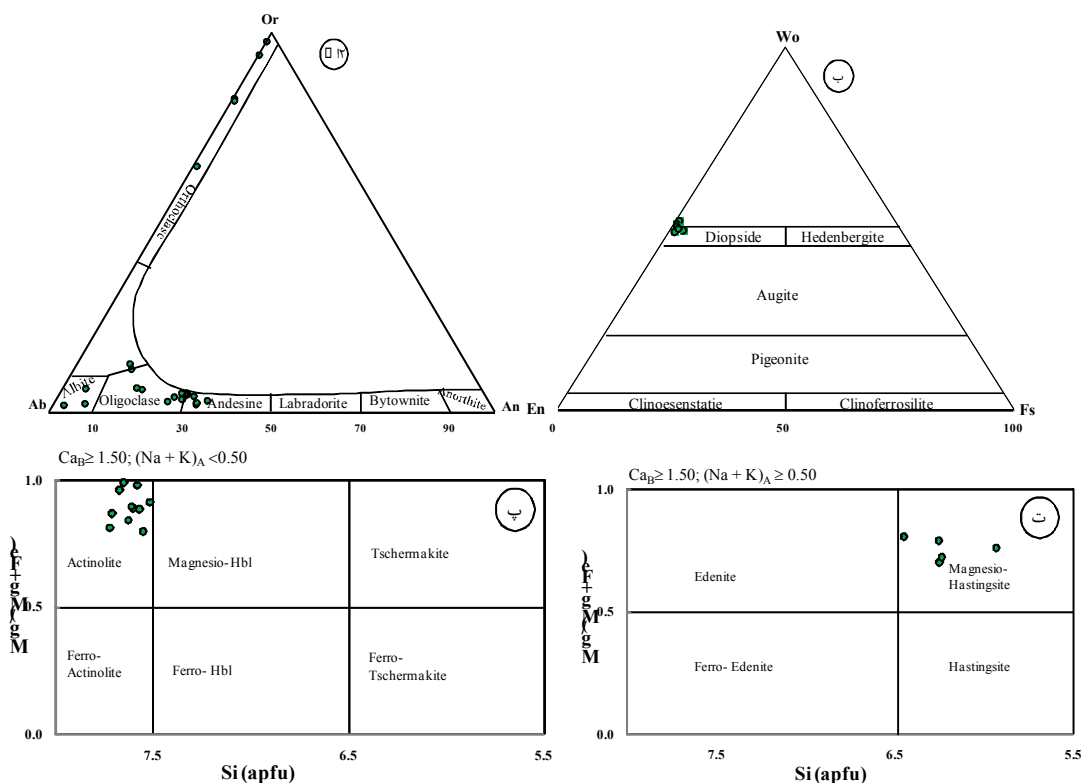
شکل ۳ نمودارهای شیمی کانی توده نفوذی منطقه اندریان (الف) نمودار مثلثی Ab-An-Or برای تعیین ترکیب پلاژیوکلازها [۲۵]، (ب) نمودار مثلثی تعیین ترکیب کلینوپیروکسن‌ها [۲۶]، (پ و ت) نمودارهای نامگذاری آمفیبول‌های کلسیمی [۲۷].
