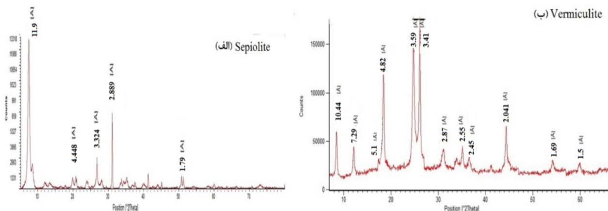
شکل ۱ پراش نگاشت پرتوی ایکس از رس‌های الف) سیپولیت و ب) ورمی کولیت.
