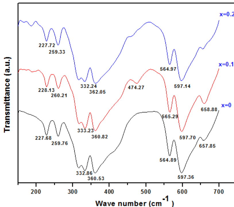
شکل ۳ طیف‌های تبدیل فوریه فروسرخ دور نمونه‌های \text{Sb}_x\text{Y}_{3-x}\text{Fe}_5\text{O}_{12} با مقادیر جانشانی (۰، ۰٫۱، ۰٫۲).
