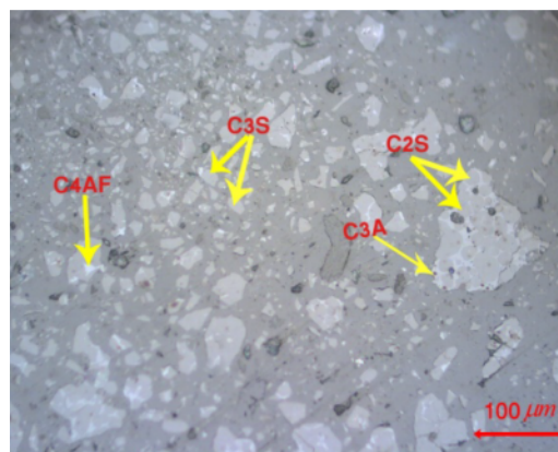
شکل ۴ مقطع صیقلی سیمان پرتلند در نور بازتابی (PPL)، دانه‌های کروی (C2S)، دانه‌های چند ضلعی (C3S)، خمیره C4AF و C3A.
