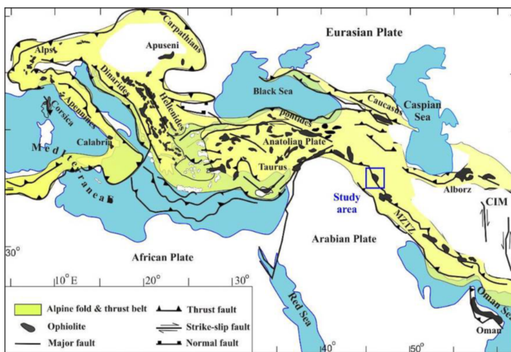
شکل ۱ توزیع همبافت‌های افیولیتی اصلی در کمربند کوهزایی آلپی [۷].
