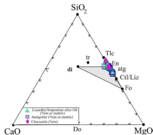
شکل ۱۳ سیستم \text{MgO-SiO}_2\text{-CaO} و نتایج تجزیه سرپانتین‌های مجموعه افیولیتی صحنه بر آن.
