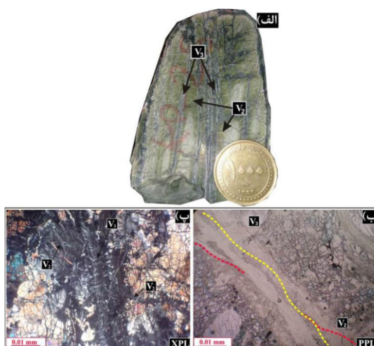
شکل ۱۱ الف- نمونه‌ای از رگه‌های نسل V_3 که رگه‌های V_2 را قطع کرده‌اند. ب، پ- نمونه‌ای از رگه‌های نسل V_3 موجود در منطقه صحنه. رگه‌های V_2 توسط رگه‌های V_3 قطع شده‌اند.
