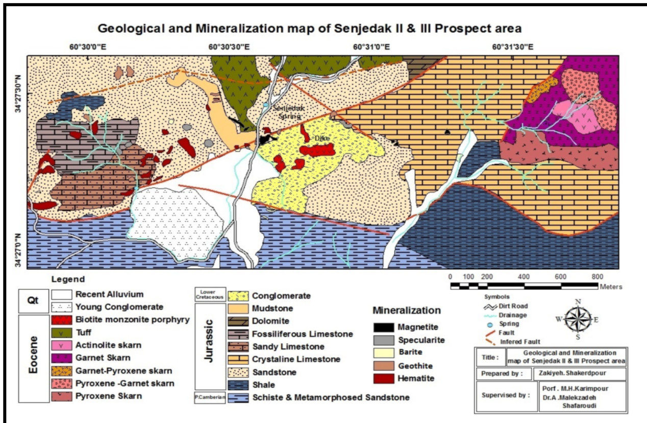
شکل ۳ نقشه‌ی زمین‌شناسی و کانی‌سازی مناطق پی‌جویی سنجدک II و III [۱۷].
